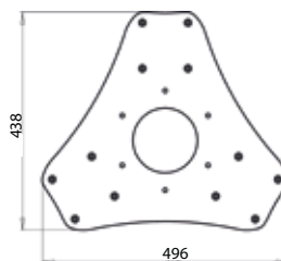
Takfäste profil
